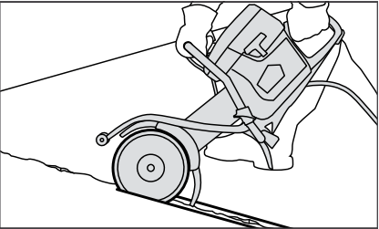
Dilatációs kapcsolatok és repedésjavítás hornyainak vágása.
