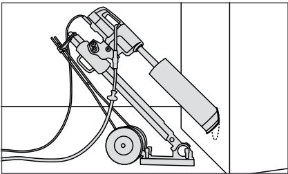
Ferde fúrás.
