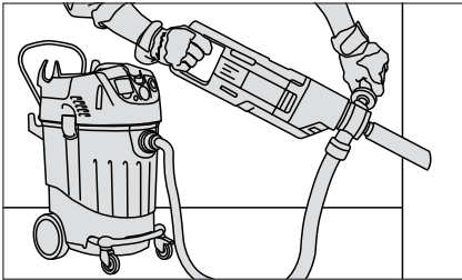
Száraz kézi fúrás.
