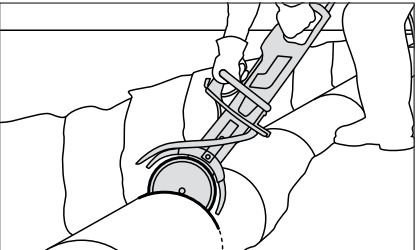
Mélyvágás csőárkokban.
