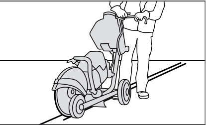
Jeltovábbító kábelek leasása.
