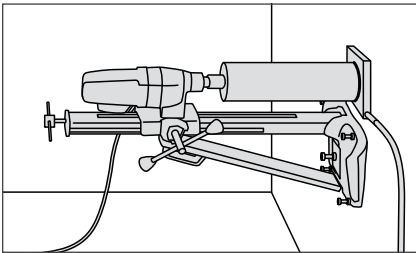
Fúrás csatornák, csövek és kábelek részére.
